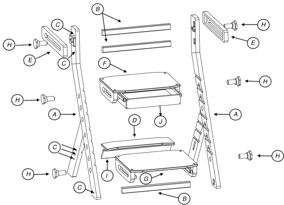
Vedere explodată – literele corespund listei de piese.
